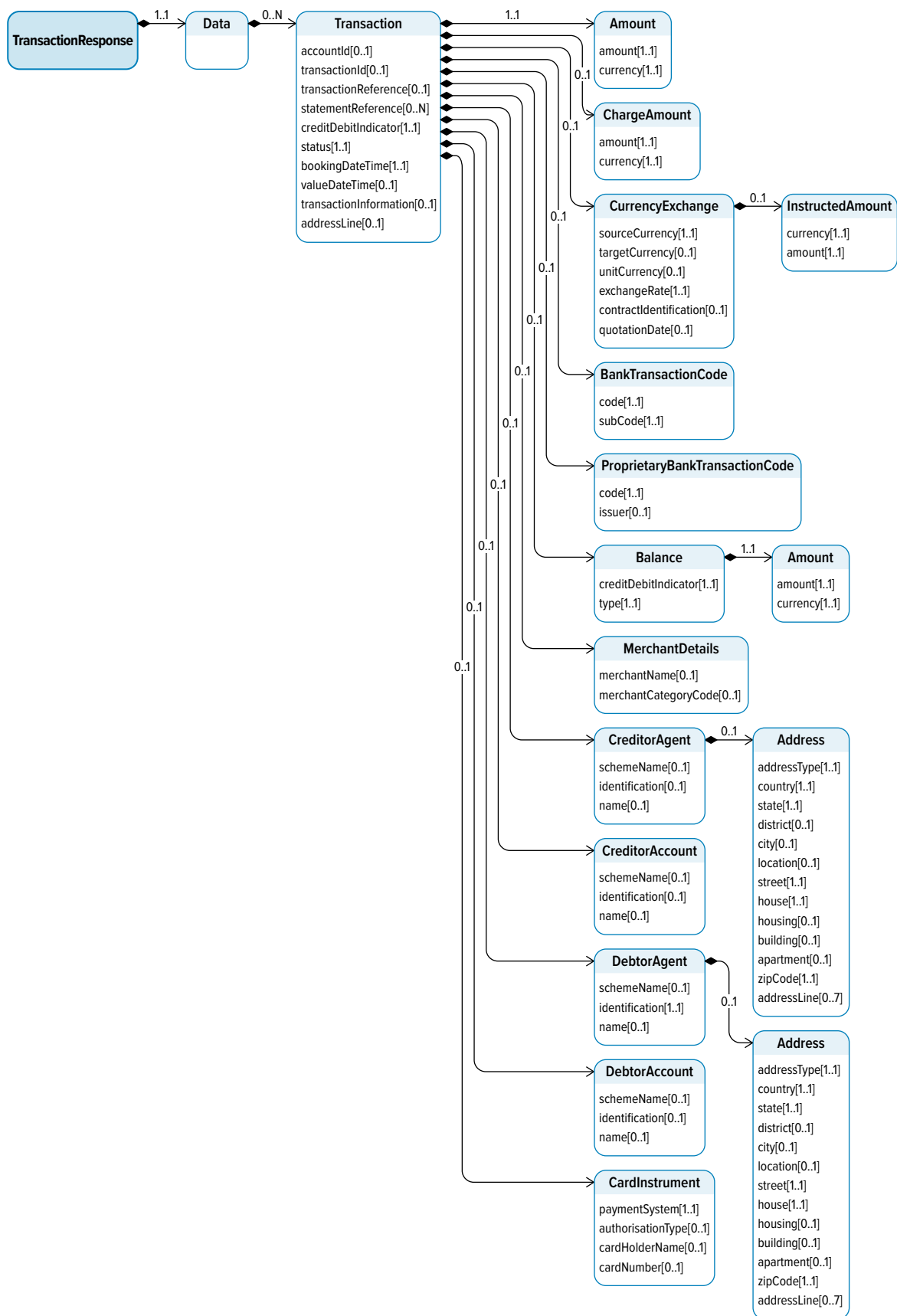
Рисунок 10. Диаграмма объекта TransactionResponse
