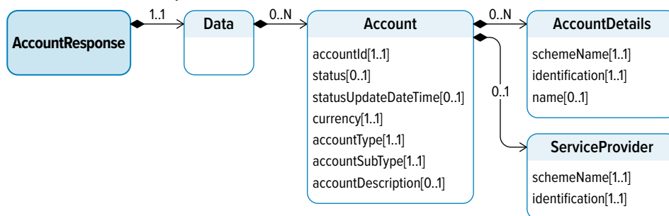
Рисунок 8. Диаграмма объекта AccountResponse
