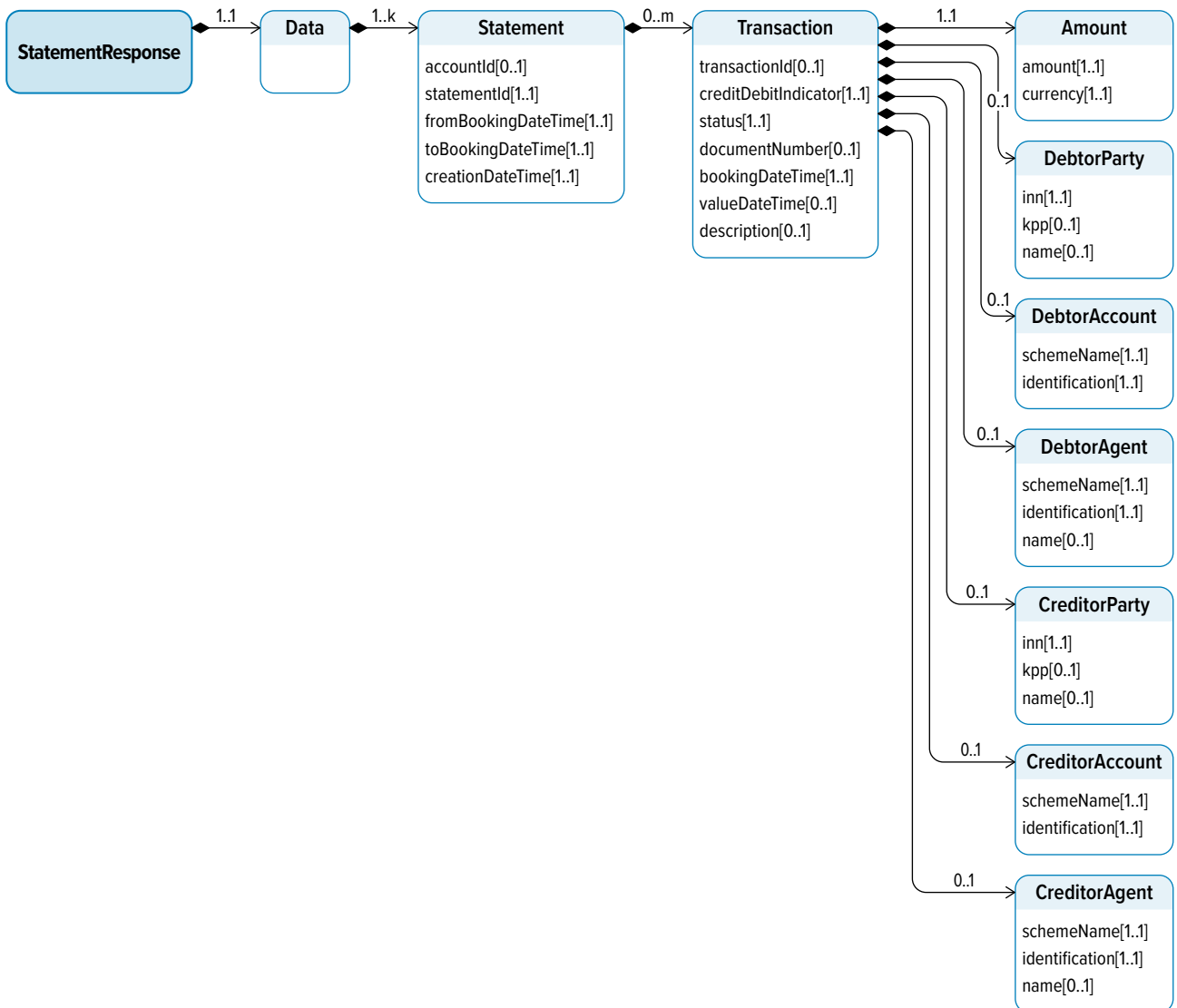
Рисунок 13. Диаграмма объекта StatementResponse
