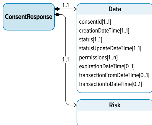
Рисунок 6. Диаграмма объекта ConsentResponse
