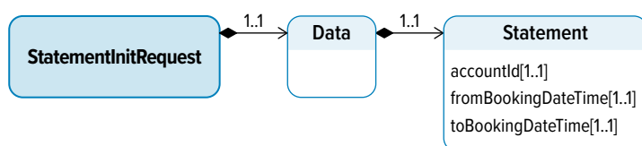
Рисунок 11. Диаграмма объекта StatementInitRequest
