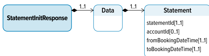
Рисунок 12. Диаграмма объекта StatementInitResponse
